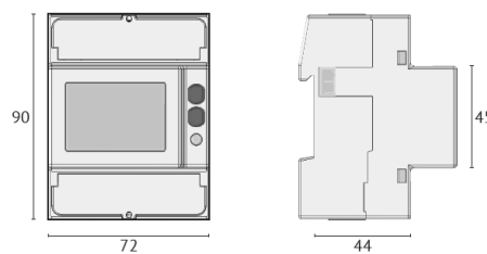
Abmessungen (mm):
